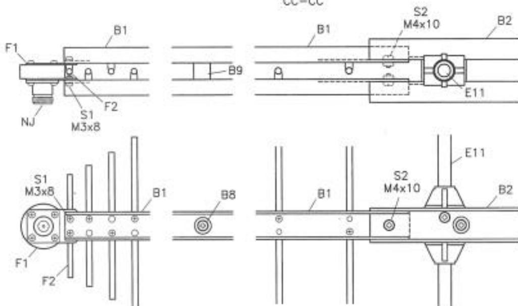
FRONT VIEW 前より見る CC-CC
