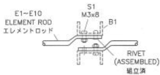
DETAIL-A 10-PLACES
