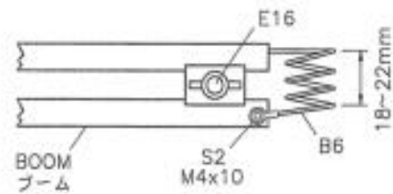
ARRESTER ASSEMBLY アレスタコイルの組立
