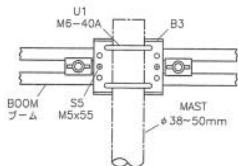
HORIZONTAL POLARIZATION 水平偏波型
